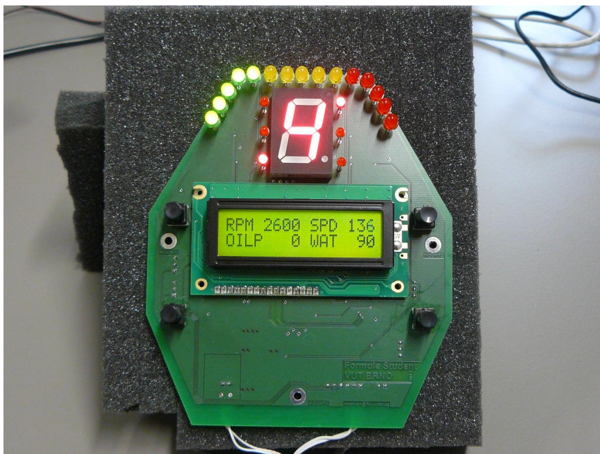
Obrázek 2 Hardware zobrazovače
